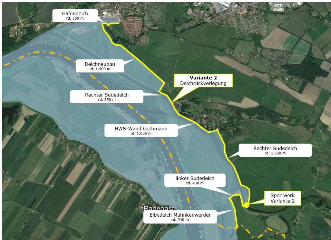
Abbildung 3-6: Variante 2 – Deichrückverlegung
