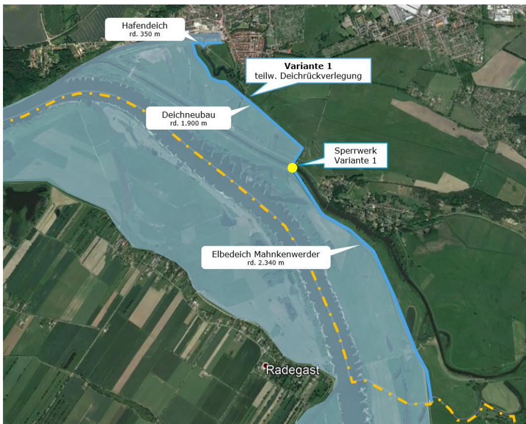
Abbildung 3-2: Variante 1 – teilweise Deichrückverlegung
