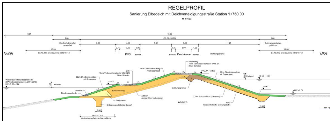
Abbildung 3-5: Regelprofil Ausbau Elbedeich
