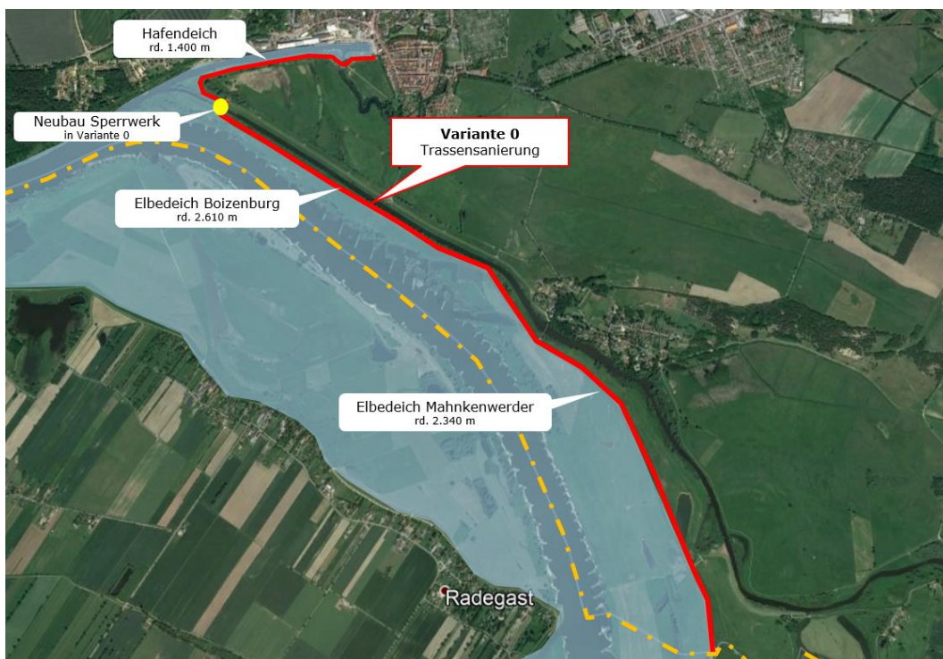
Abbildung 3-4: Variante 0: Sanierung in der Trasse
